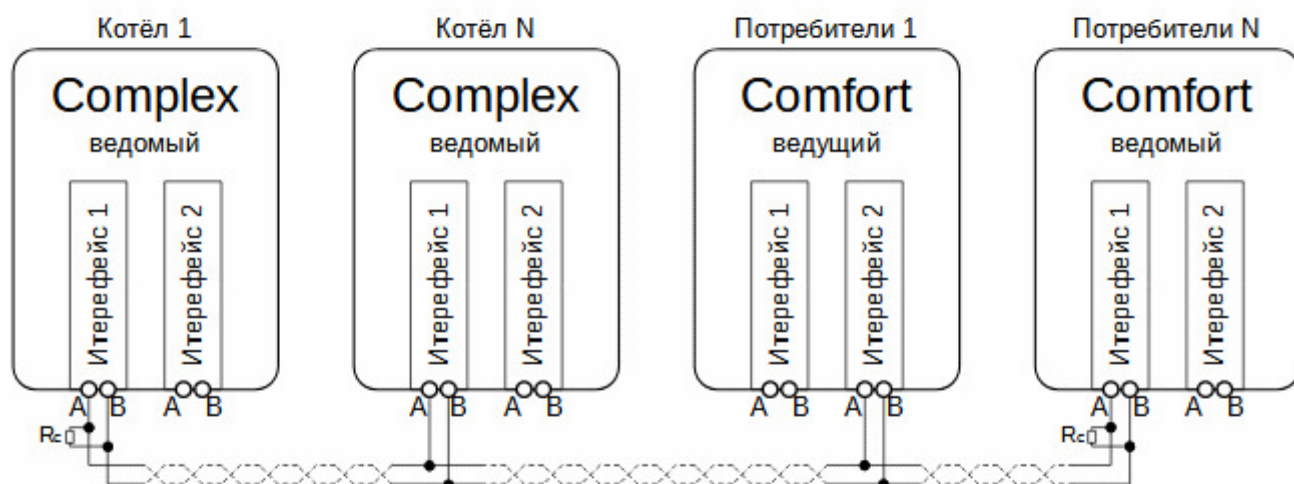
Вариант 2. Пульт Comfort — ведущий в системе каскада котлов.
