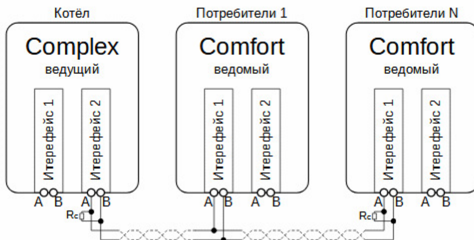
Вариант 3. Пульт Complex — ведущий в системе с одним котлом.
