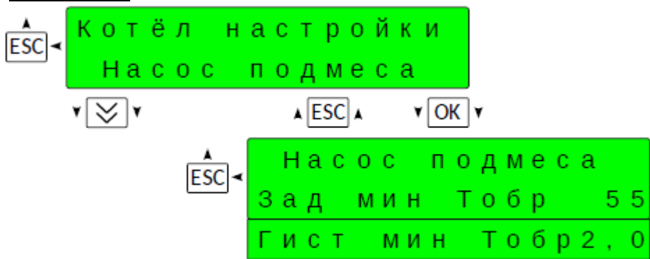
Рисунок 10 – Меню «Настройки котел» / Подменю «Насос подмеса»
